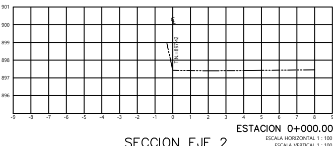
SECCION EJE 2
