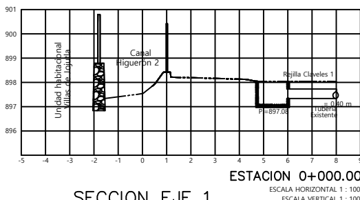
SECCION EJE 1
